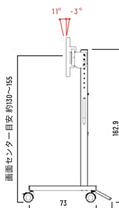
モニター側面図
