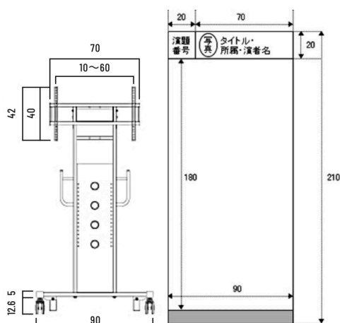
ポスター、モニター台正面図
